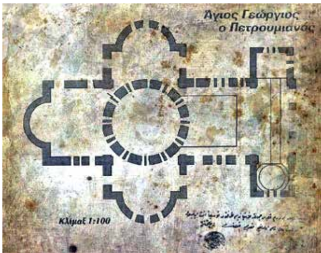
Το σχέδιο της κάτοψης του υπό ανέγερση νέου ναού του Αγ. Γεωργίου στην Αλικαρνασσό. (Αρχείο Μιχ. Τριανταφύλλου)
